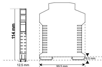
TxIsoRail-HART
